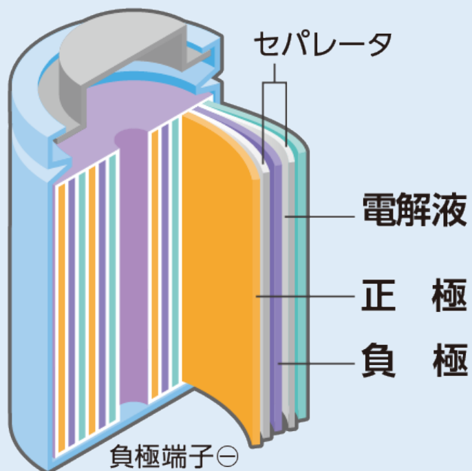
リチウムイオン電池 (円筒型) 正極端子⊕
